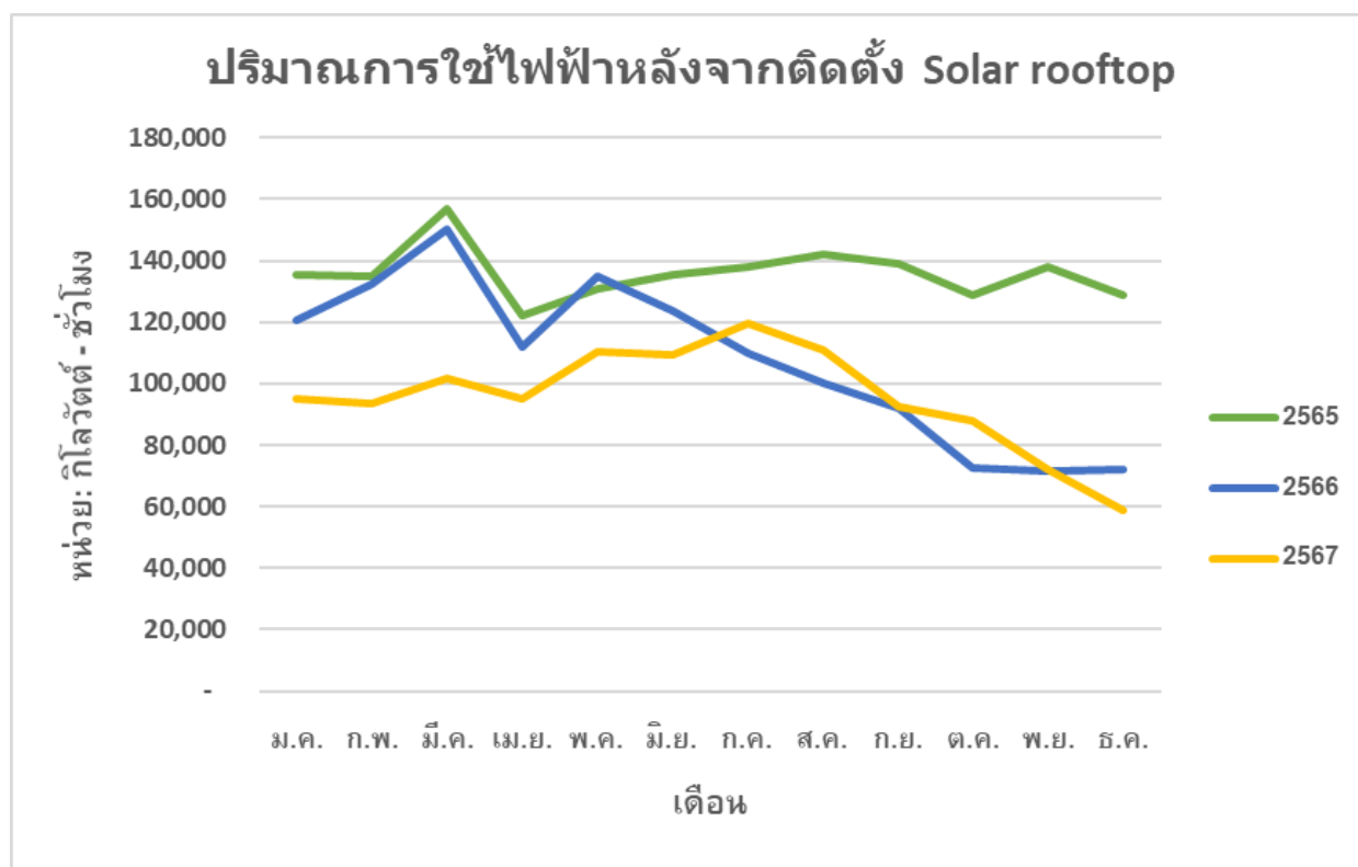
ปริมาณการใช้ไฟฟ้าหลังติดตั้ง Solar rooftop
